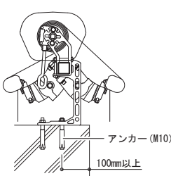
▼RC造 納まり
