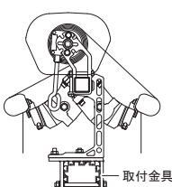
▼アルミ取付枠 納まり
