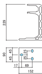
▼取付ブラケット 寸法図
